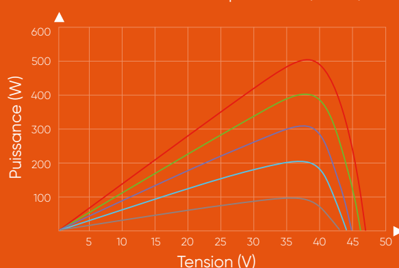
Courbe de tension & puissance (500W)
