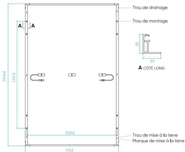
Vue arrière - dimensions en mm
